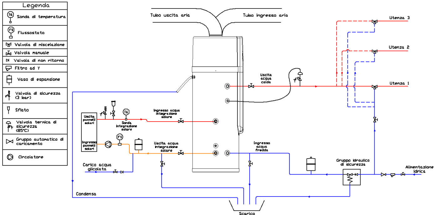
Schema di installazione in caso di ricircolo di acqua di integrazione solare
