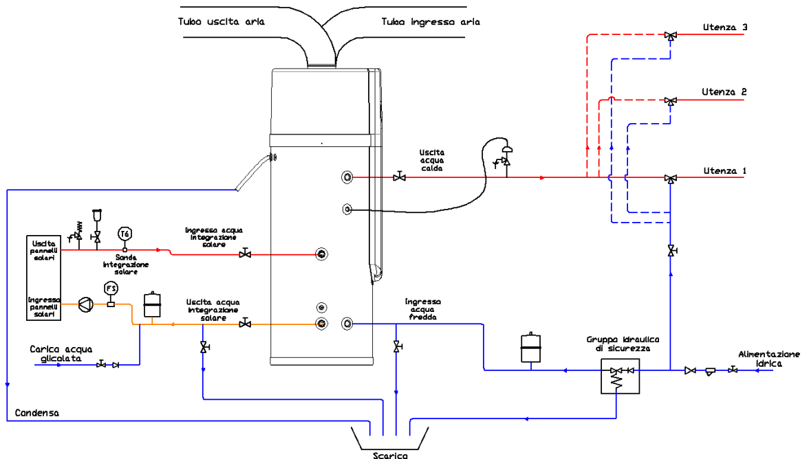
Schema di installazione in caso di ricircolo di acqua di integrazione solare Nota: il serpentino di integrazione solare è presente solo sui modelli UNICA S1 e UNICA S2
