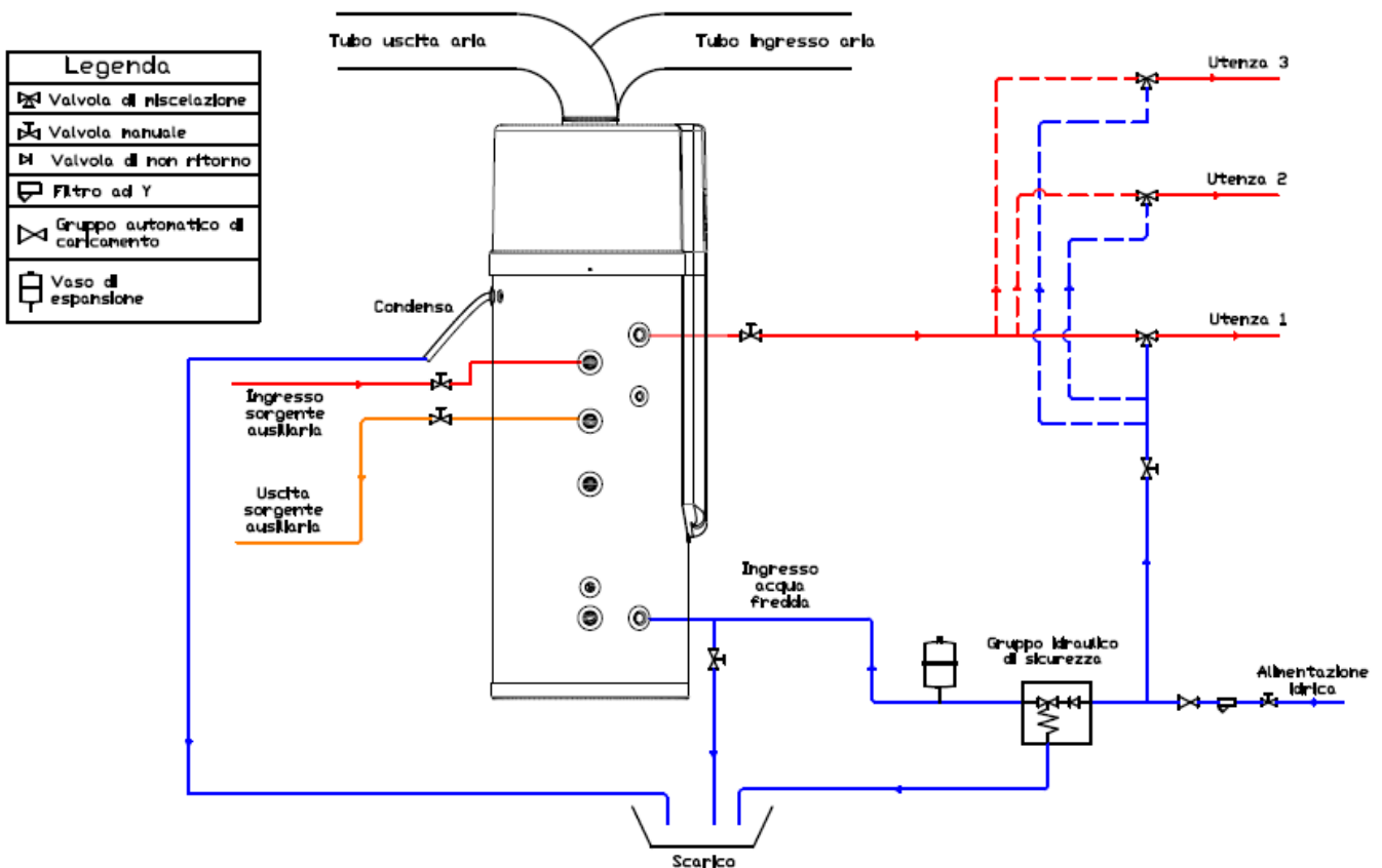
Schema di installazione in caso di fonte di calore ausiliaria Nota: il serpentino di integrazione ausiliario è presente solo nei modelli UNICA S2
