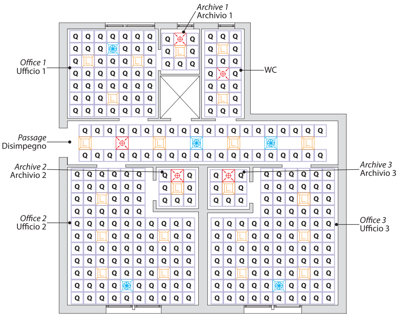
Positioning of the radiant panels Disposizione dei pannelli radianti
