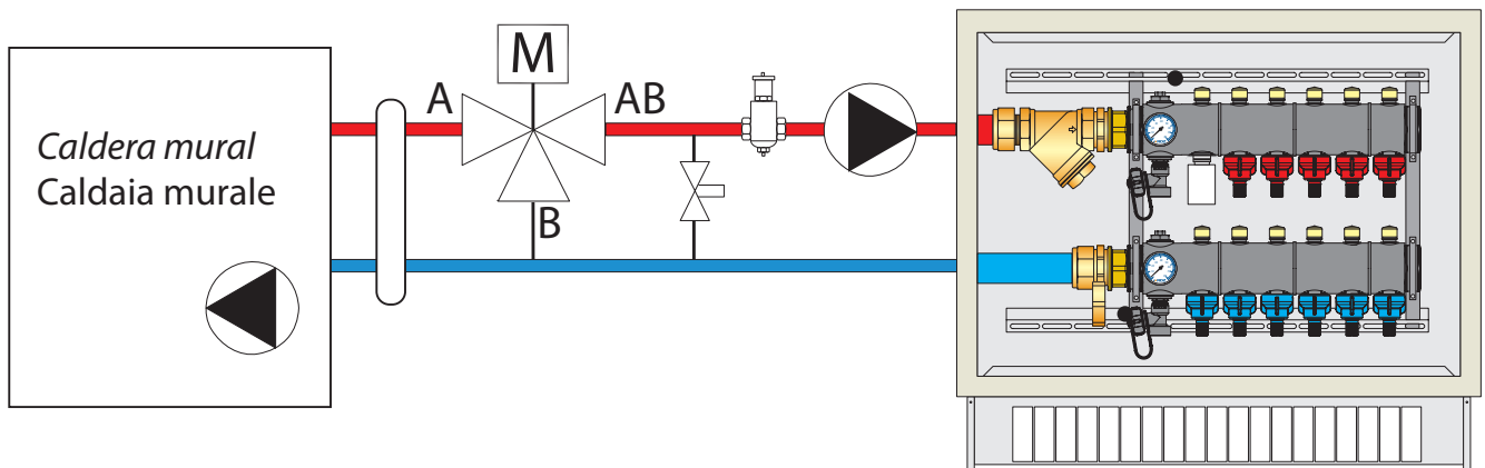
Esquema hidráulico indicativo de la instalación de calefacción con sistema b!klimax Schema idraulico indicativo di principio dell'impianto di riscaldamento con sistema b!klimax
