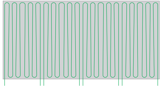
1200x600 mm Circuito/Circuito 12 m 2 circuitos elemental 2 circuiti elementari
