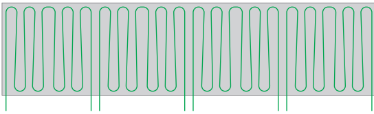
600x600 mm Circuito/Circuito 6 m 4 circuitos elemental 4 circuiti elementari
