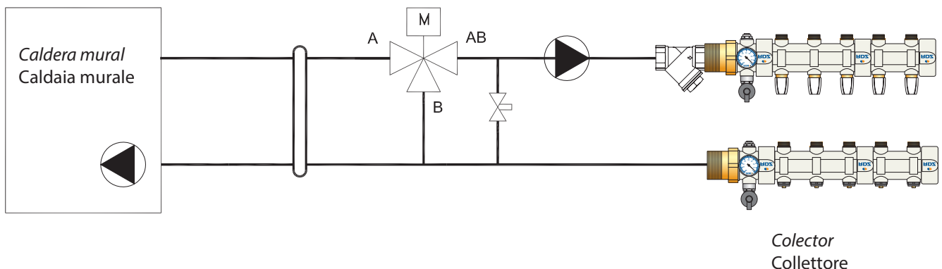
Esquema hidráulico indicativo de la instalación de calefacción con sistema b!klimax Schema idraulico indicativo di principio dell'impianto di riscaldamento con sistema b!klimax
