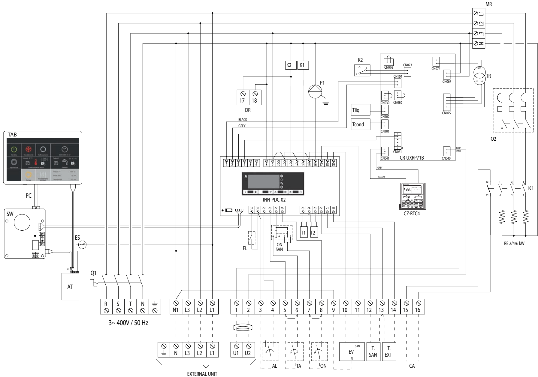
2.10.9 Schema elettrico trifase con resistenze e web server (v. legenda pag. 23)
