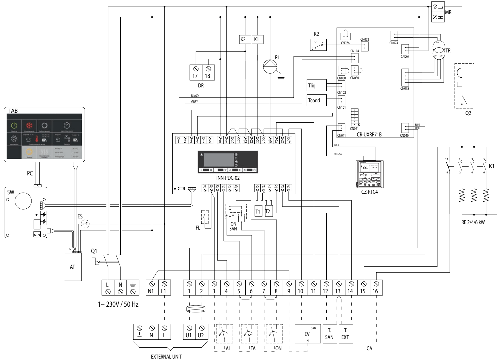
2.10.5 Schema elettrico monofase con resistenze e web server (v. legenda pag. 23)
