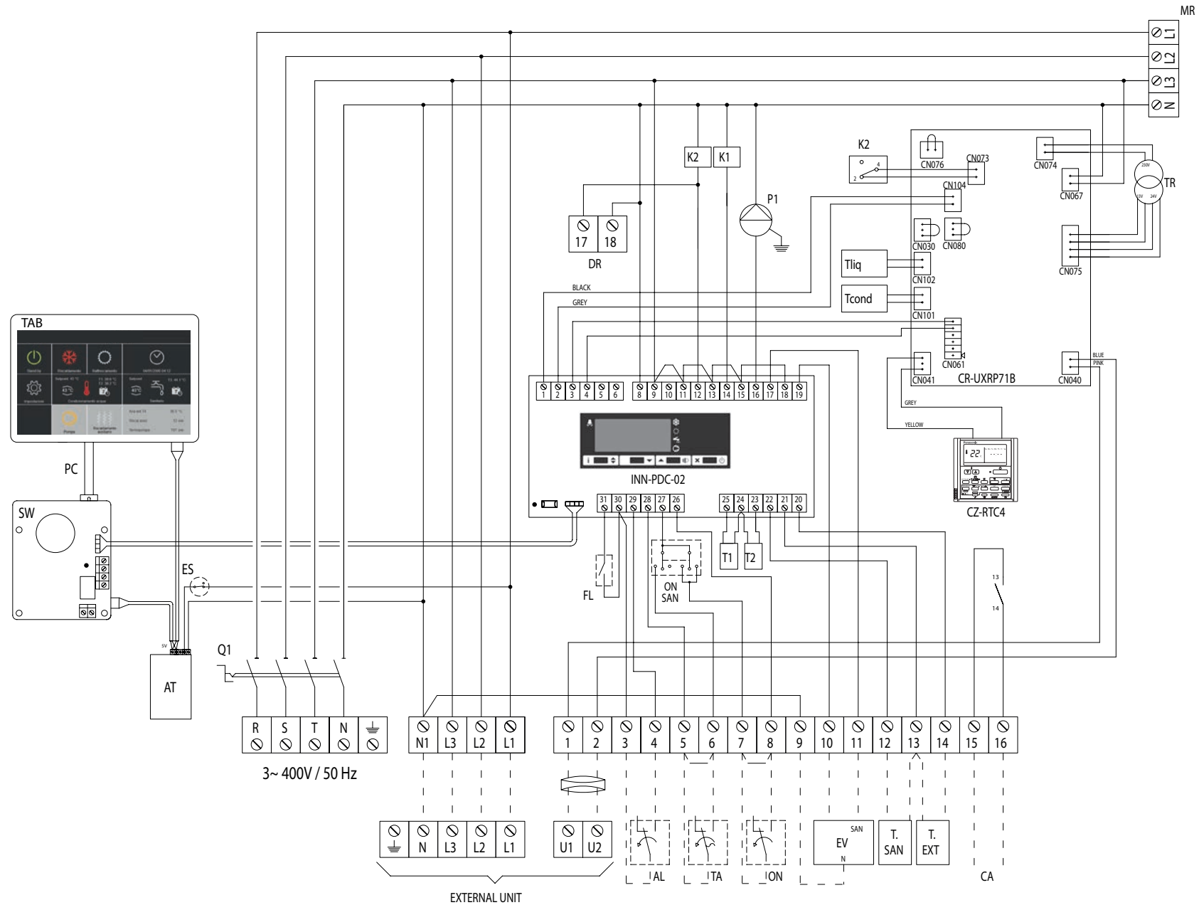
2.10.8 Schema elettrico trifase con web server Raspberry (v. legenda pag. 23)
