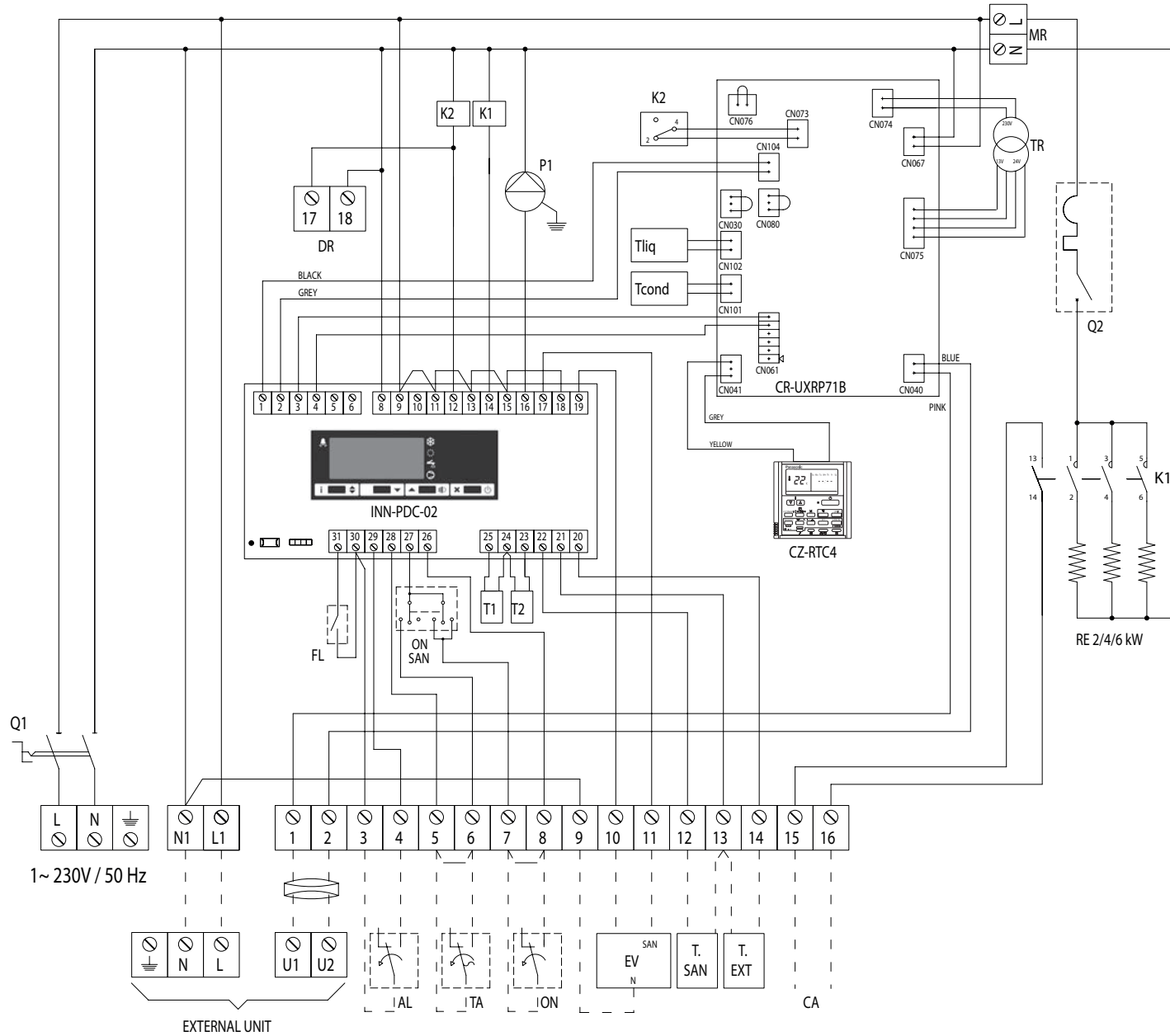
2.10.3 Schema elettrico monofase con resistenze (v. legenda v. pag. 23)
