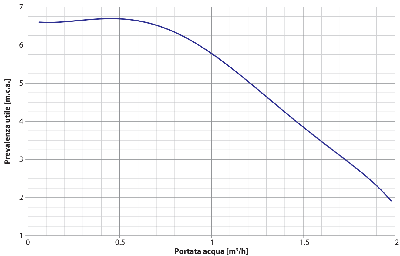
GM 3 PUNTI DN 25
