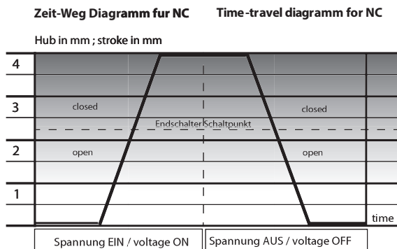
Zeit-Weg Diagramm für NC mit Endschalter Time-travel diagram for NC with Endswitch Hub in mm; stroke in mm
