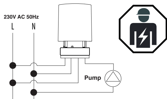
Anschlusschema Wiring diagram Hub in mm; stroke in mm
