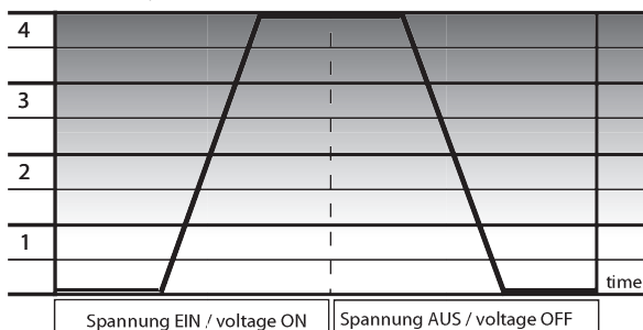
Zeit-Weg Diagramm für NC Time-travel diagram for NC
