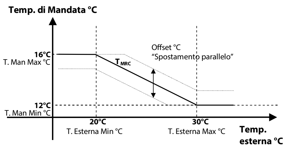
Curva di Raffrescamento (compensazione Estiva).
