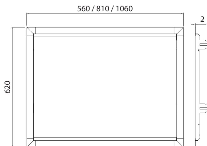
Frame (smooth version) Telaio a filo per armadietto Slim
